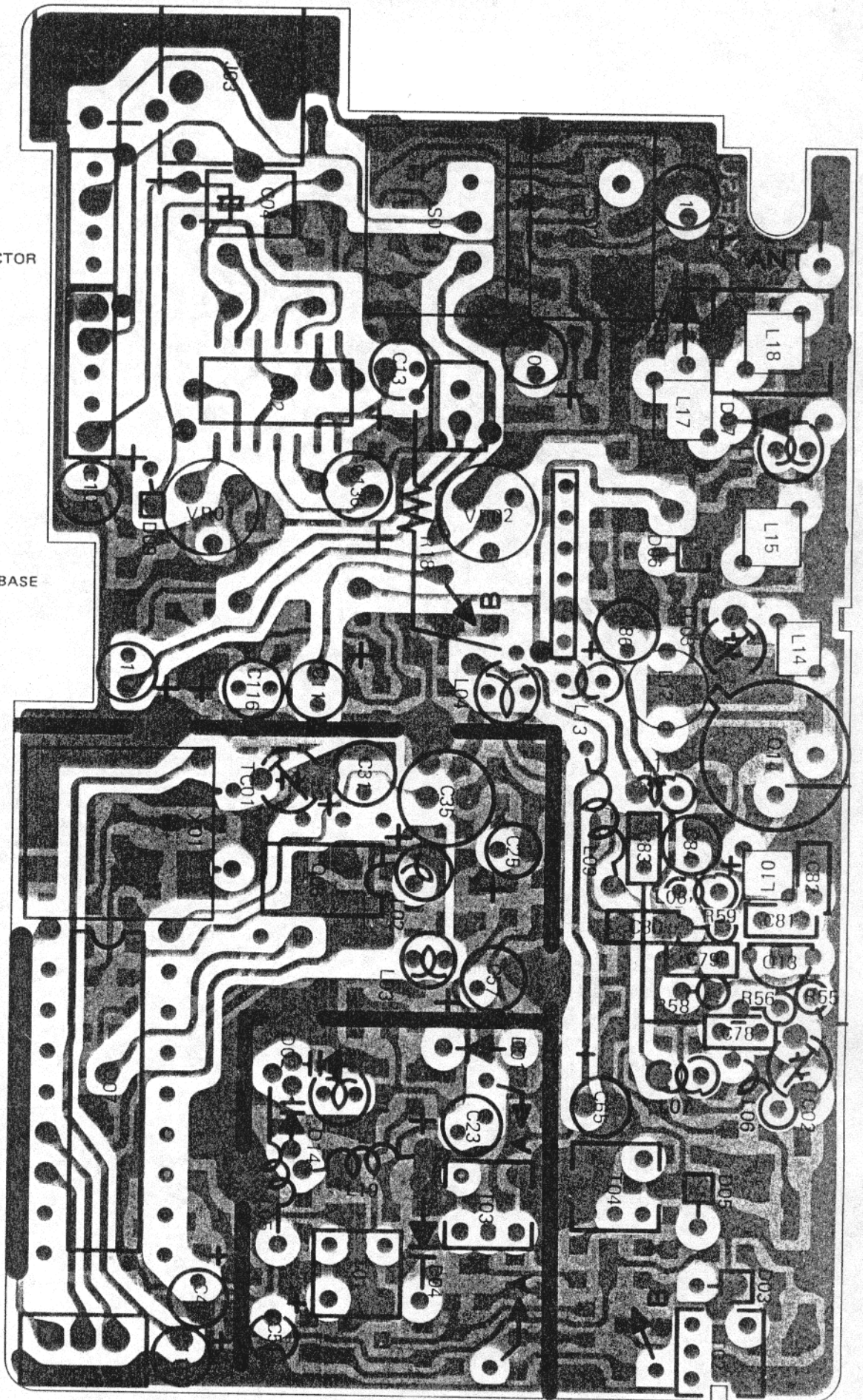
2SC1947 (Q2014)
